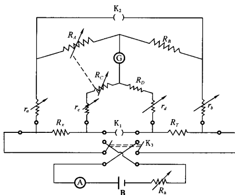
图 1 三次平衡双电桥原理线路图
