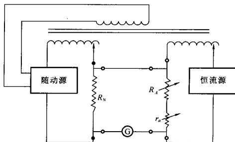
图 5 电流比较仪电桥检定测量盘线性度误差的原理线路图
